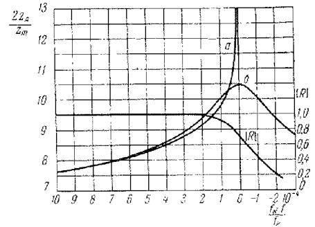
Рис. 33,6. Высотно-частотная характеристика и коэффициент отражения |R| для параболического слоя ( z_m = 12 км, \lambda_k = 30 м): a — приближение геометрической оптики; b — строгое решение.
