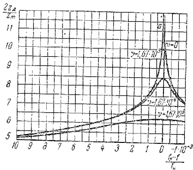
Рис. 33.8. Высотно-частотные характеристики для параболического слоя ( z_m = 36 км, \lambda_k = 90 м) при различных значениях \nu_{эфф} = \nu . Кривая a — приближение геометрической оптики при \nu = 0 ; все остальные кривые — точные решения.
