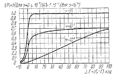
Рис. 33.4. Коэффициент отражения при z_m = 6 км и \lambda_k = 90 м.
