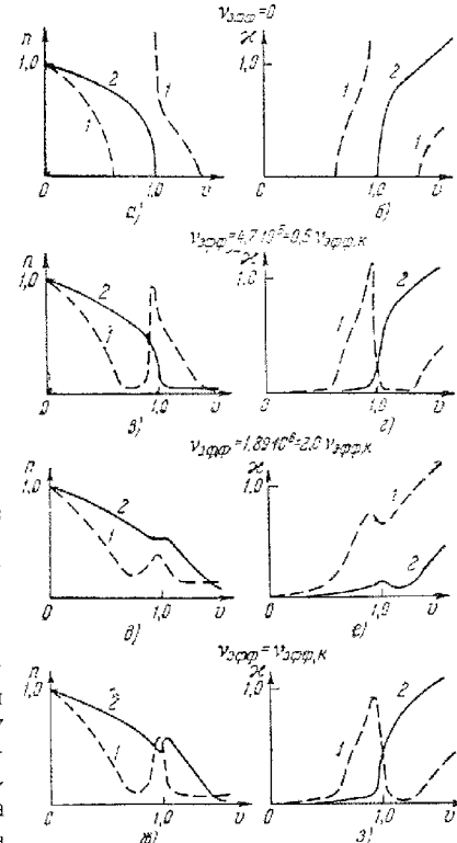
Рис. 11,13. Показатели преломления и поглощения для \lambda = 80 м и различных значений v_{эфф} (значения \alpha и u = \frac{\omega_H^2}{\omega^2} указаны в тексте; пунктир относится к волнам типа 1, сплошные линии — к волнам типа 2).
