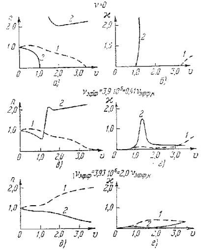
Рис. 11,15. Показатели преломления и поглощения для \lambda = 490 м и различных значений \nu_{эфф} (значения а и б указаны в тексте).
