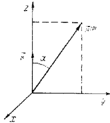
Рис. 11,1. Координатная система, используемая в § 11.
