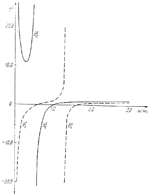
Рис. 11,7. Функции \tilde{n}_{1,2}^2\left(\frac{\omega}{\omega_0}\right) при \frac{\omega_H}{\omega_0} = 1 , \alpha = 45^\circ .
