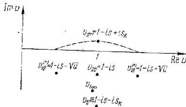
Рис. 28,4. Комплексная плоскость переменной v .
