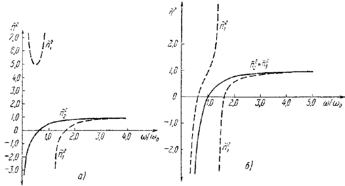
Рис. 11.5. а — функции n_{1,2}^2\left(\frac{\omega}{\omega_0}\right) = 1 - \frac{1}{\left(\frac{\omega}{\omega_0}\right)\left(\frac{\omega}{\omega_0} \pm \frac{\omega_H}{\omega_0}\right)} , отвечающие
