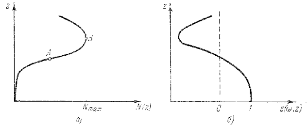
Рис. 30.4. Произвольный плавный слой с одним максимумом.
