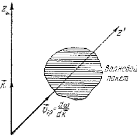
Рис. 12,5. Движение волнового пакета.
