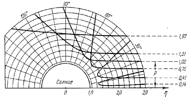
Рис. 36,2. Траектории лучей в солнечной короне для радиоизлучения с длиной \lambda_0 = 5 м. На рисунке указаны значения «прицельного параметра» p , выраженного в единицах радиуса фотосферы r_\odot .
