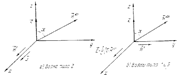
Рис. 14.1. Волны типа 1, 2 и 3 в магнитной гидродинамике.
