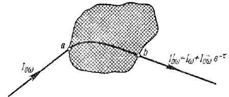
Рис. 36,8. Изменение интенсивности излучения при прохождении луча через поглощающую среду.
