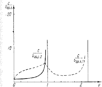
Рис. 35,4. Отношение скорости света к проекции групповой скорости на ось z (нормаль к слою) в зависимости от \nu = \frac{\omega_0^2}{\omega^2} . Значения \alpha и u указаны в тексте.
