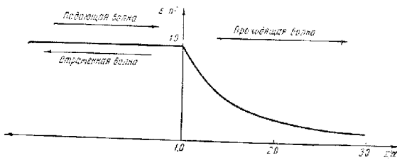
Рис. 17,3. Слой \varepsilon = \frac{a^2}{z^2} при \frac{z}{a} > 1 .
