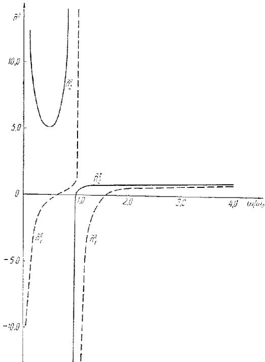
Рис. 11,11. Функции \tilde{n}_{1,2}^2\left(\frac{\omega}{\omega_0}\right) при \frac{\omega_H}{\omega_0} = 1 и \alpha = 10^\circ .
