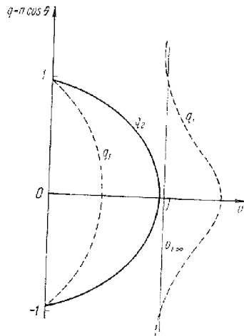
Рис. 29,2. Функции q_{1,2}(v) для распространения на полюсе (вертикальное магнитное поле H^{(0)} ). Используются значения \theta_0 = 20^\circ , u = \frac{1}{4} .
