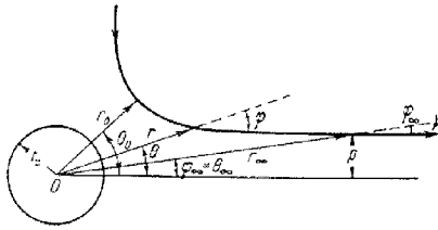
Рис. 36,1. Траектория луча в солнечной короне.
