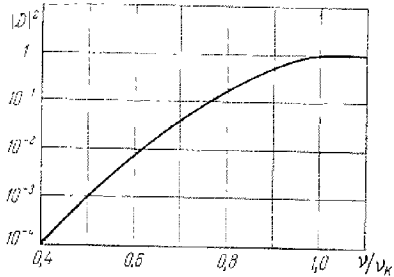
Рис. 28,8. Коэффициент пропускания |D|^2 как функция \frac{\nu}{\nu_k} при u = \frac{1}{4} и \omega = 1,76 \cdot 10^7 ( \lambda_0 = 107 м). Кривая рассчитана для параболического слоя ( z_m = 30 км) при \nu_k = \frac{\omega_H \sin^2 \alpha}{2 \cos \alpha} = 2,3 \cdot 10^5 ; критическая частота для волны 2 f_{k2} \equiv f_{k0} = 4 мГц, f = 3,47 мГц, f_H = \frac{\omega_H}{2\pi} = 1,44 мГц и \alpha = 13^\circ .
