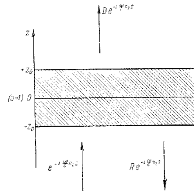
Рис. 28.3. Отражение от слоя неоднородной плазмы при u \ll 1 .
