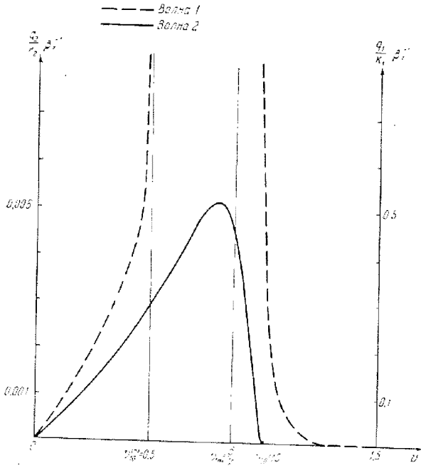
Рис. 12,6. Величины \frac{q_{1,2}}{k_{1,2}} \beta_T^{-1} в зависимости от \nu = \frac{\omega_0^2}{\omega^2} при
