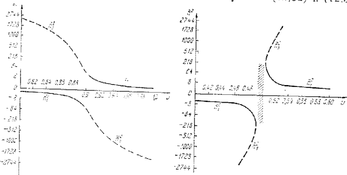
Рис. 12,8. Функции \tilde{n}_1^2 и \tilde{n}_3^2 при u = 0,1 , \alpha = 90^\circ и \beta_T^2 = 10^{-5} . По оси ординат на рис. 12,8—12,12 используется логарифмический масштаб.
