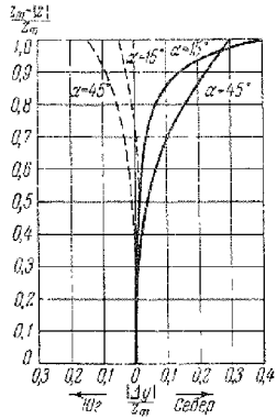
Рис. 35,2. Отклонение лучей от вертикали при нормальном падении для \alpha = 15^\circ и \alpha = 45^\circ при f_H = 1,4 мггц. Обыкновенный луч (сплошные линии) f = f_{к0} = 9 мггц, необыкновенный луч (пунктир) f = f_{кx} \approx 9,75 мггц.
