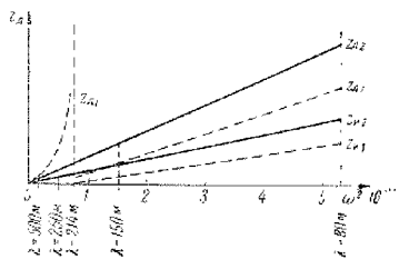
Рис. 35,5. Действующая высота отражения z_x и истинная высота отражения z_n для линейного ионосферного слоя в зависимости от частоты \omega . Пунктир относится к волне типа 1, а сплошные линии — к волне типа 2 (обыкновенной).
