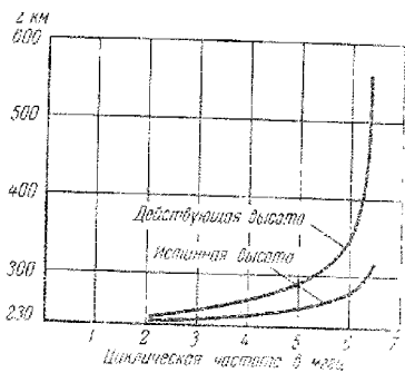
Рис. 30.6. Действующая (кажущаяся) и истинная высота отражения для F_2 -слоя.
