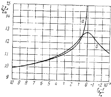
Рис. 33,5. Высотно-частотная характеристика для параболического слоя ( z_m = 120 км, \lambda_k = 30 м) вблизи критической частоты: a — приближение геометрической оптики; b — строгое решение.
