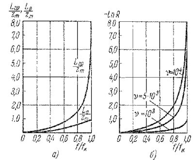
Рис. 31.1. а — значения \frac{L_{\text{гр}}}{z_m} и \frac{L_0}{z_m} для параболического слоя как функции \frac{f}{f_k} ; б — логарифм коэффициента отражения для параболического слоя при z_m = 100 км как функция \frac{f}{f_k} для среднего эффективного числа соударений \nu_{\text{эфф}} = 10^3, 5 \cdot 10^3 и 10^4 .
