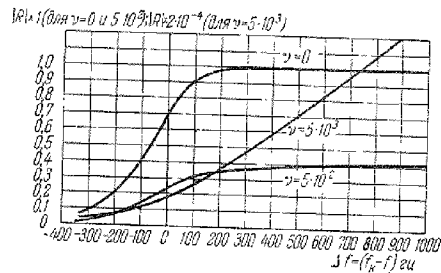
Рис. 33.3. Коэффициент отражения |R|^2 для параболического слоя z_m = 120 км, \lambda_k = \frac{c}{f_k} = 30 м при различных значениях числа соударений \nu_{эф} \equiv \nu .
