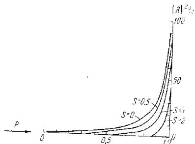
Рис. 18,4. Коэффициент отражения для «переходного» слоя.
