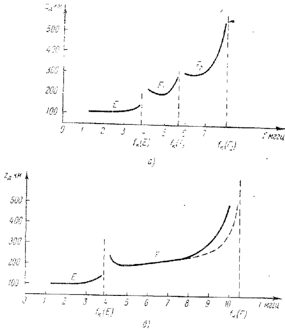
Рис. 30,5. Высотно-частотные характеристики ионосферы (схематически): а — летом и б — зимой.
