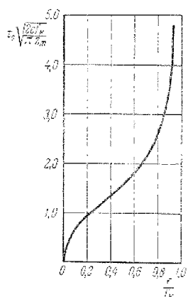
Рис. 30,7. Время установления \tau_0 (умноженное на \sqrt{\frac{2cf_k}{\pi z_m}} ) для параболического слоя.
