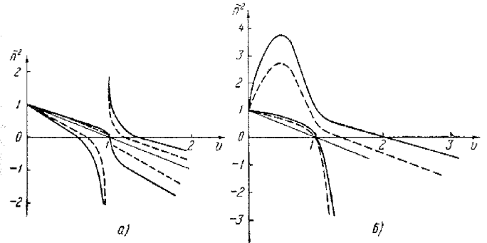
Рис. 11,16. Квадрат показателя преломления в случае смеси электронов и ионов \xi = \frac{N_i m}{N M} , где N и N_i — концентрации электронов и ионов, а m и M — их массы: а) \lambda = 80 м; б) \lambda = 225 м. Жирная линия: \xi = 0 , тонкая линия: \xi = \infty , пунктир: \xi = 1 .
