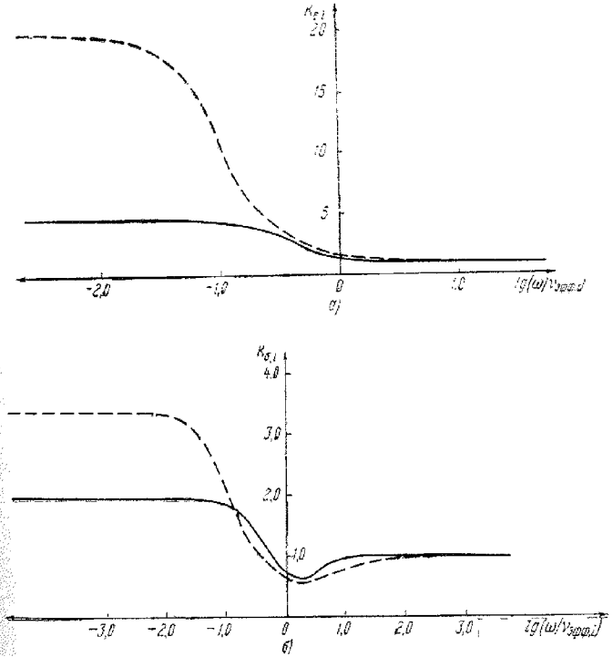
Рис. 6,2. Функции K_{\epsilon, l} \left( \frac{\omega}{v_{эфф, l}} \right) и K_{\sigma, l} \left( \frac{\omega}{v_{эфф, l}} \right) . Сплошные кривые — при учете междуэлектронных соударений, пунктирные линии — без учета междуэлектронных соударений (по оси абсцисс отложен десятичный логарифм \frac{\omega}{v_{эфф, l}} ).
