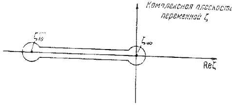
Рис. 27,4. Контур интегрирования в выражении (27,17), причем контур нужно обойти два раза (двулистый характер поверхности на рисунке не отражен).
