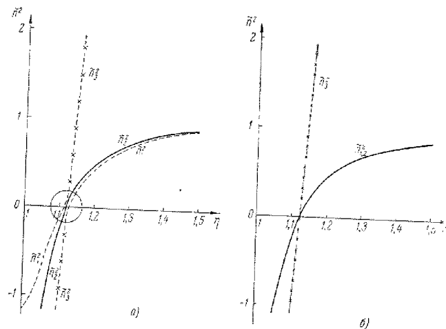
Рис. 36.7. Функции \tilde{n}_{1,2,3}^2 в корональной плазме при \alpha = 15^\circ : а) H_0 = 25 эрст; б) H_0 = 0 (изотропная плазма).
