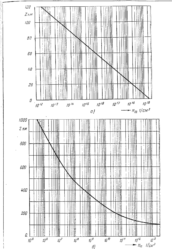
Рис. 30,2. Концентрация нейтральных частиц (молекул) N_m в атмосфере: а — высоты, меньше 120 км; б — высоты, больше 100 км.
