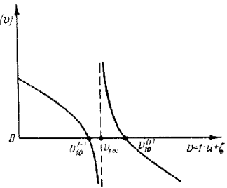
Рис. 27,3. Функция \tilde{n}_1^2(v) при a = \frac{\pi}{2} .
