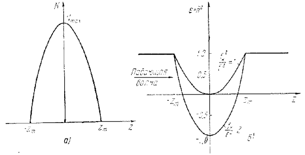
Рис 17,2. Параболический слой: а) N(z) ; б) \epsilon(z) при \frac{f_k^2}{f^2} = 1 и \frac{f_k^2}{f^2} = 2 .
