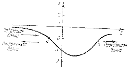
Рис. 33,2. Диэлектрическая проницаемость \varepsilon для плавного слоя с одним максимумом.
