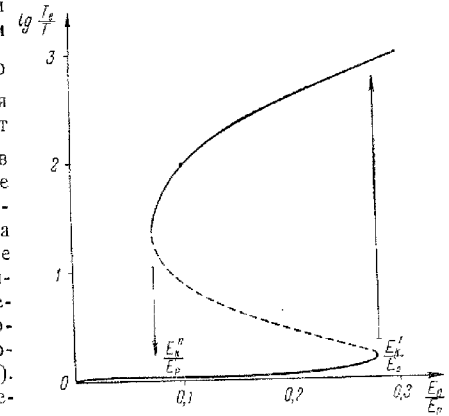
Рис. 38,2. Зависимость электронной температуры от напряженности электрического поля в случае соударений электронов с ионами ( \omega = 0,01\nu_0 ).
