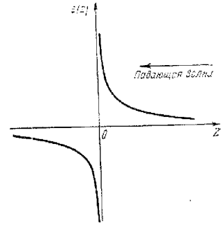
Рис. 27,1. Слой \varepsilon(z) = \frac{g^2}{z} .
