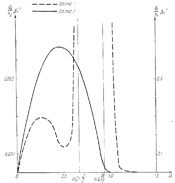
Рис. 12,7. Величины \frac{q_{1,2}}{k_{1,2}} \beta_T^{-3} в зависимости от \nu = \frac{\omega_0^2}{\omega^2} при
