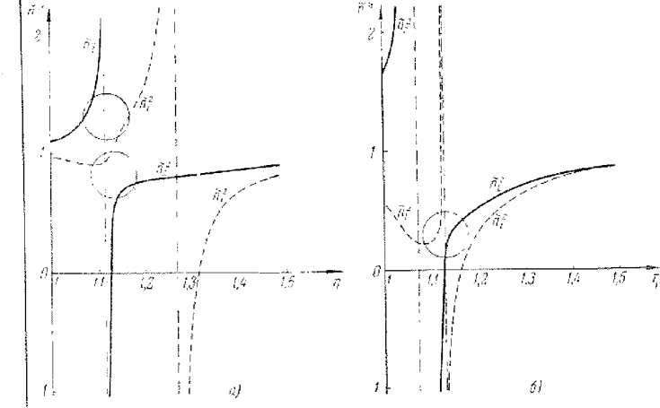
Рис. 36,5. Функции \tilde{n}_{1,2}^2(\eta) в корональной плазме при \alpha = 15^\circ (вертикальные пунктирные линии отвечают точкам \omega_{1\infty} и \omega_{2\infty} ): а) H_b = 2,5 \cdot 10^3 ; б) H_b = 2,5 \cdot 10^2 .
