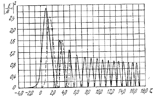
Рис. 32,1. Структура поля вблизи точки отражения (сплошная линия). Пунктиром нанесено отношение \left| \frac{E}{A} \right|^2 в приближении геометрической оптики (32,7). Параметр \zeta = \left\{ \frac{\omega^2}{c^2} \left| \frac{d\varepsilon}{dz} \right|_0 \right\}^{1/2} \Delta z .
