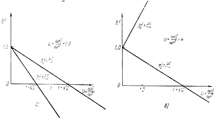
Рис. 11,2. Функции \tilde{n}_{1,2}^2(\nu) \equiv \tilde{n}_{\pm}^2(\nu) при u = \text{const} в случае продольного распространения (т. е. при \alpha = 0 ): а) u < 1 ; б) u > 1 .
