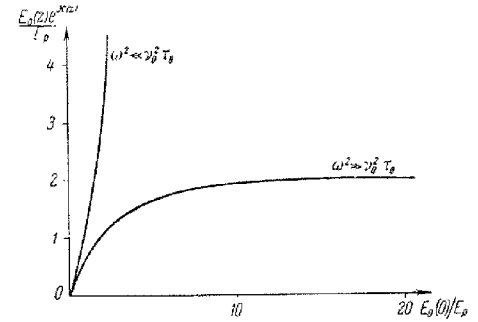
Рис. 39,1. Зависимость \frac{E_0(z) e^{\mathcal{K}(z)}}{E_p} от \frac{E_0(0)}{E_p} (соударения с молекулами).
