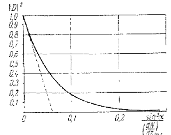
Рис. 28,7. Коэффициент пропускания |D|^2 как функция от \frac{\sin^2 \alpha}{\left(\frac{dN}{dz}\right)_{v=1}}
