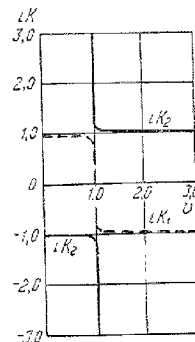
Рис. 11,12. Отношение полюсов iK_{1,2} при \alpha = 10^\circ и u = \frac{1}{4} .
