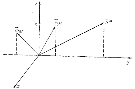
Рис. 24.1. Направление векторов групповой скорости v_{гр1,2} .
