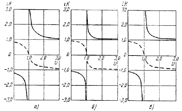
Рис. 11.9. Отношение полуосей эллипса поляризации iK_1 (пунктир) и iK_2 (сплошные линии): а) u = \frac{1}{4} , \alpha = 45^\circ ; б) u = 1,08 , \alpha = 20^\circ ; в) u = 4 , \alpha = 20^\circ .
