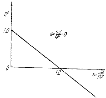
Рис. 11,4. Функция \tilde{n}_{1,2}^2(\nu) \equiv \tilde{n}_0^2(\nu) для изотропной плазмы.
