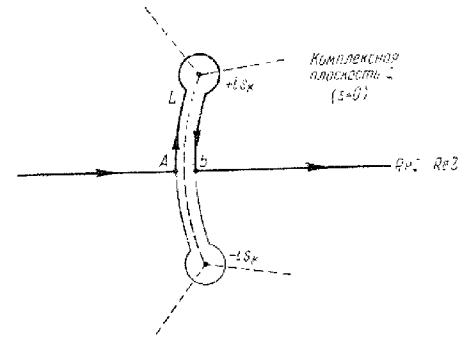
Рис. 28,5. Контур интегрирования в выражении (28,45).
