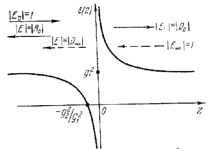
Рис. 27,2. Слой \varepsilon(z) = g_1^2 + \frac{g_2^2}{z} .
