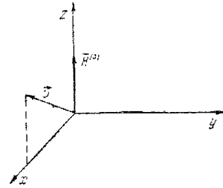
Рис. 13,1. Координатная система, используемая при записи соотношений (13,34), (13,37) и (13,38).
