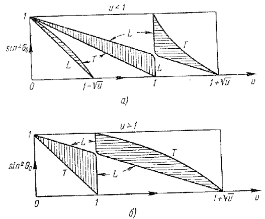
Рис. 29.6. Области изменения нулей функций q_{1,2}(v) : а) u = \frac{1}{4} ; б) u = 4 .
