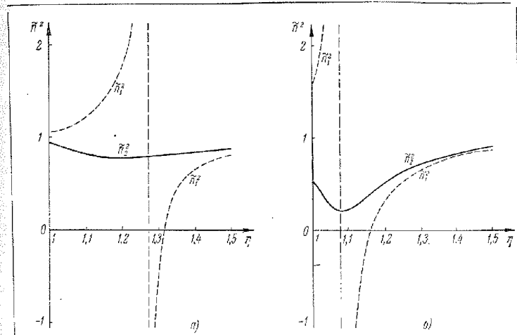
Рис. 36,4. Функции \tilde{n}_{1,2}^2(\eta) в корональной плазме при \alpha = 0 (вертикальные пунктирные линии отвечают точке \omega_{1\infty} ): а) H_b = 2,5 \cdot 10^3 ; б) H_b = 2,5 \cdot 10^2 .
