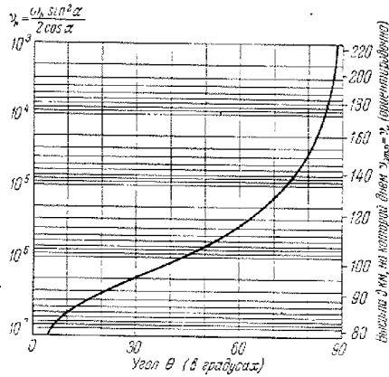
Рис. 28,6. Критическое число соударений \nu_k в зависимости от геомагнитной широты \theta . Справа даны высоты, для которых по грубо ориентировочным данным \nu_{эфф} = \nu_k при f_H = 1,44 мгц.
