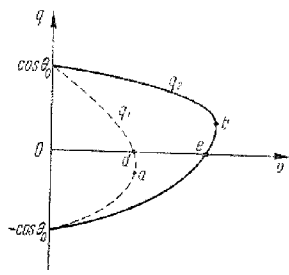
Рис. 29.5. Схематический вид функций q_{1,2}(v) при u < 1 (проведена лишь одна ветвь кривой q_1(v) ).
