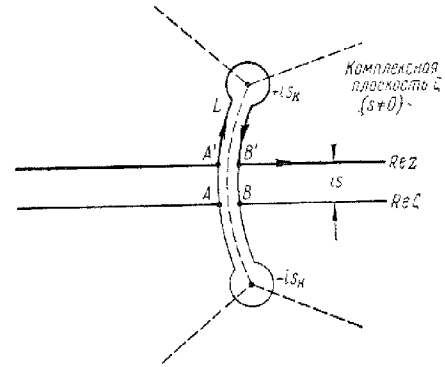
Рис. 28,9. Контур интегрирования в выражении (28,53).
