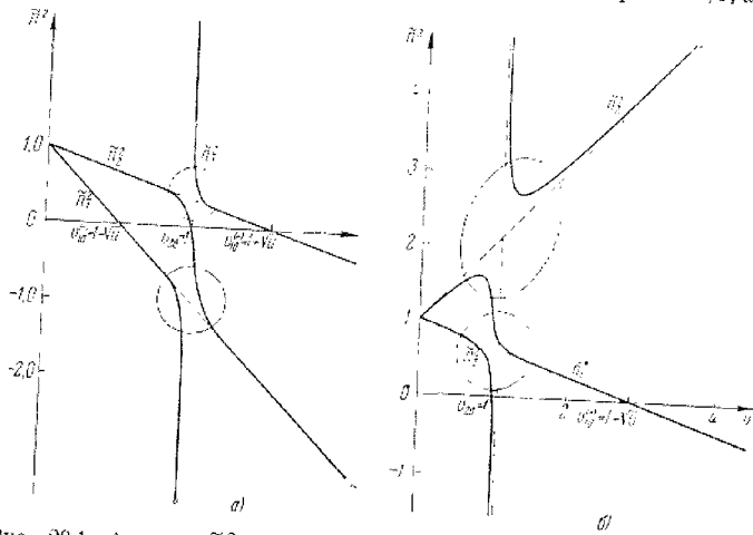
Рис. 28.1. Функции \tilde{n}_{1,2}^2 при малых углах \alpha (схематический рисунок; пунктир относится к углу \alpha = 0 ): а) u < 1 ; б) u > 1 .
